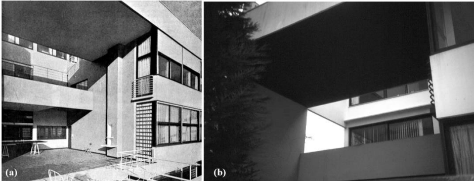
Figura 8: Espacio exterior recortado de la Villa Stein (Le Corbusier, 1927). Fuente: Boesiger & Stonorov (1970, t.1: 149); y fotografía propia.
