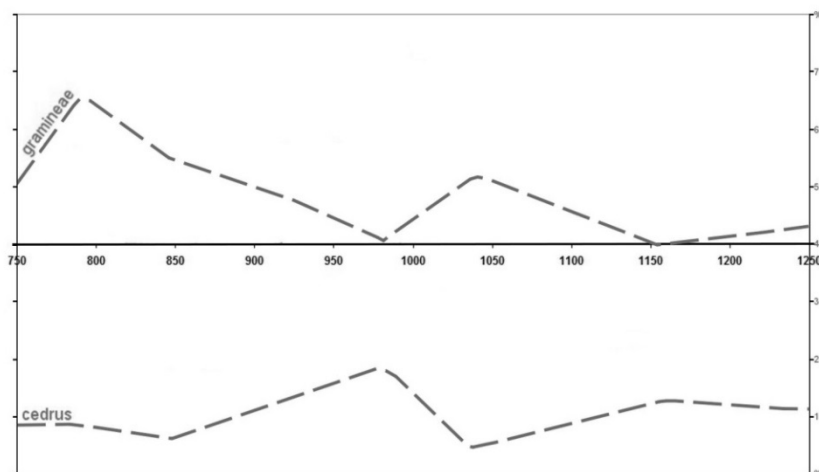
Figura 7. Índices polínicos registrados de Cedrus atlantica y gramineae en el lago Tiguilmamine. Los valores representan el porcentaje recogido en la muestra C86 (De: LAMB, H. F. et al., “Relations between century-scale”. p. 137, fig. 2).
