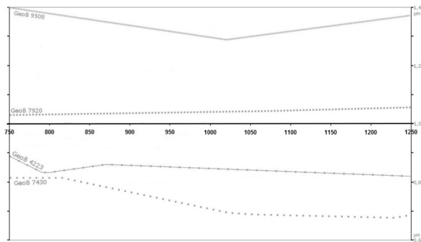
Figura 10. Biomarcadores sobre las aportaciones fluviales recogidos en los sondeos marinos GeoB 4223; GeoB 7430; GeoB 7920 y GeoB 9508 (De MEYER, I. et al., “Grain size control” y MEYER, I. et al. “Changing rainfall patterns in NW Africa”).
