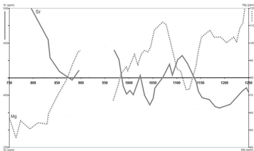
Figura 8. Concentraciones de estroncio (Sr) y magnesio (Mg) en la estalagmita GP5 de la Gruta del Piste. Existe un hiato entre los años 900 y 975 (De: WASSENBURG, J. A. et al., “Moroccan speleothem”, p. 295, fig. 5).
